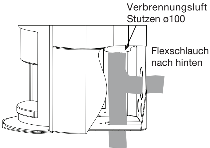
Flex-Schlauch durch den Boden
