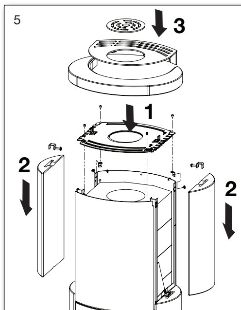
Montage von Steinen. Stellen Sie die Seiten und die Oberseite ein.
